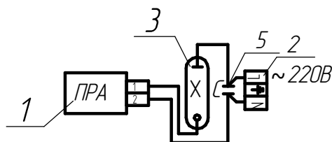
ПКУ Схема №1
