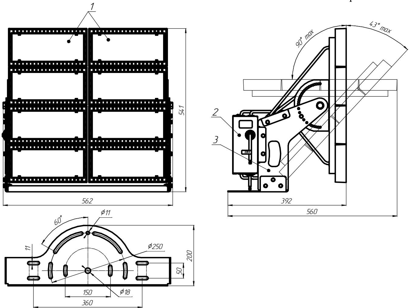
Рисунок 1 - Внешний вид и габариты прожекторов серии ДО16
