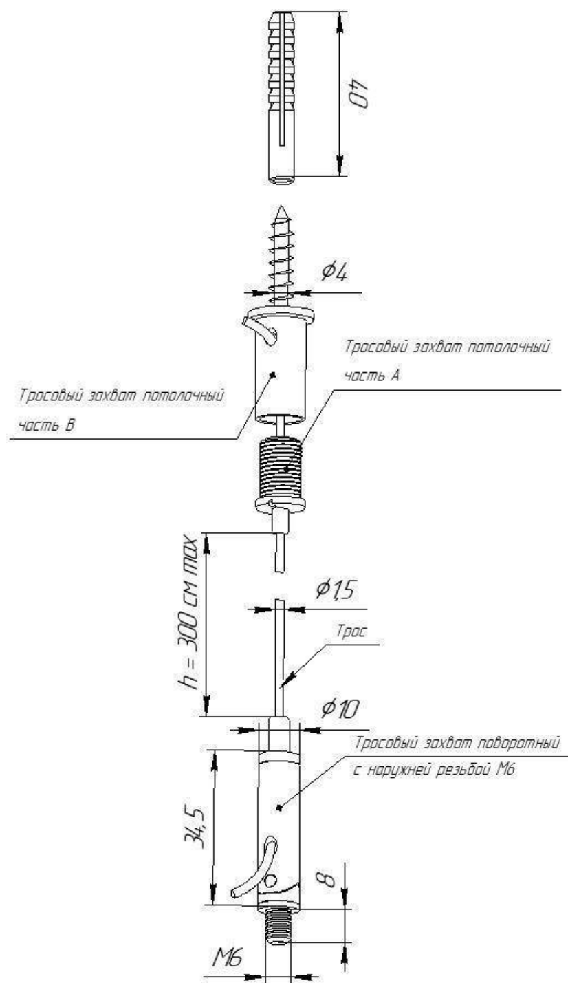
Рисунок 7 - Сборка тросового подвеса
