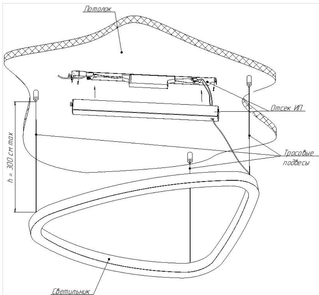
Рисунок 6 - Схема установка светильников
