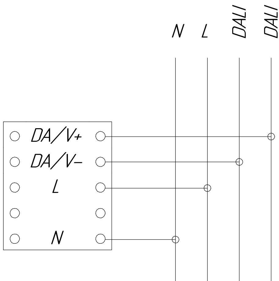
Рисунок 3а - Схема подключения светильников для модификаций -001, -031
