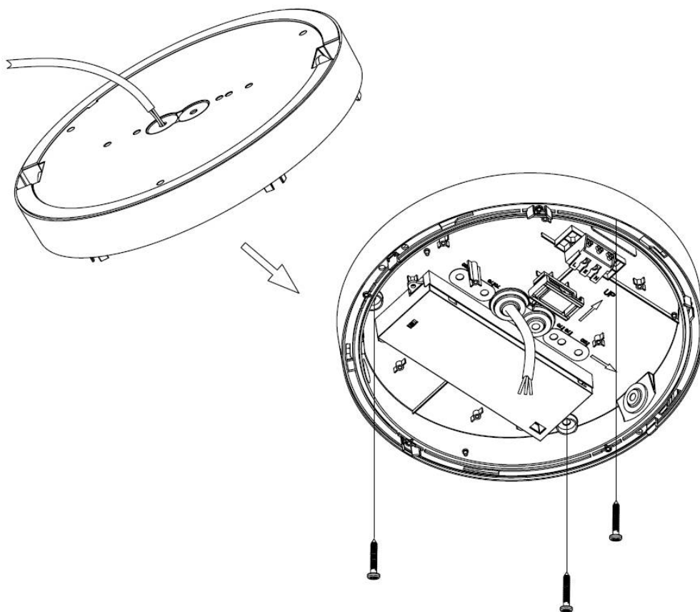
Рисунок 2в - Установка светильника на рабочую поверхность
