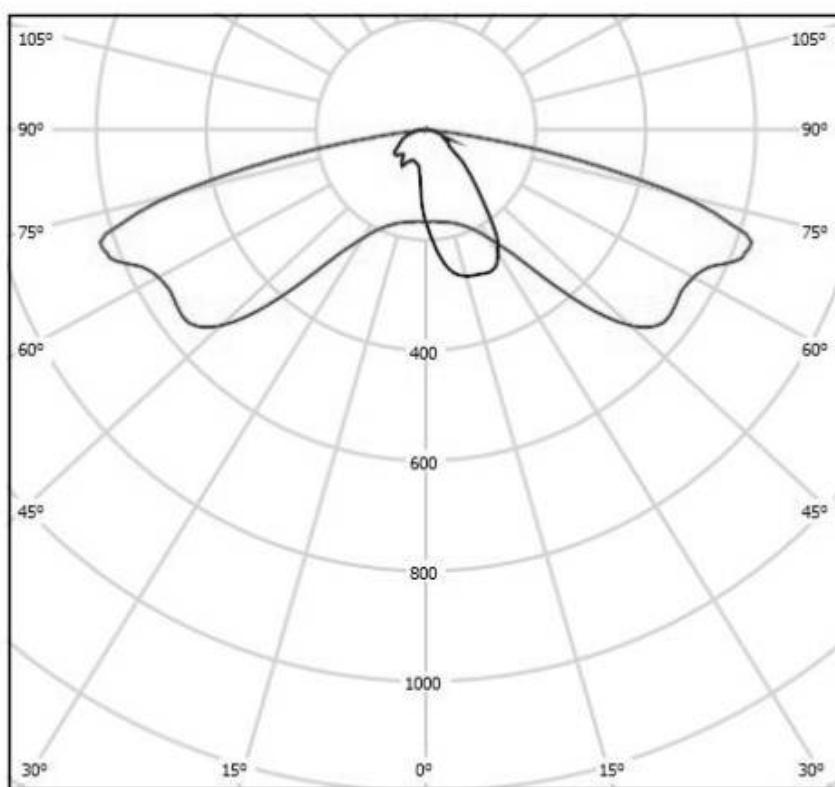
Рисунок 4 - Кривая силы света.
