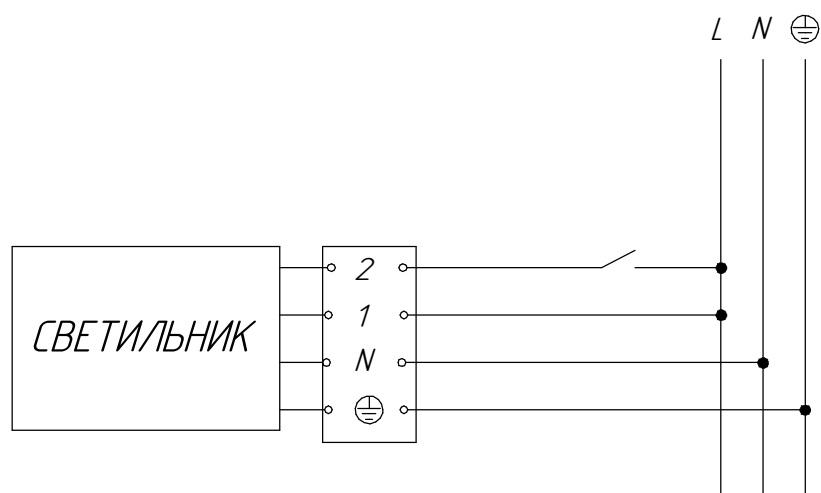
Рисунок 4 - Схема подключения светильников
