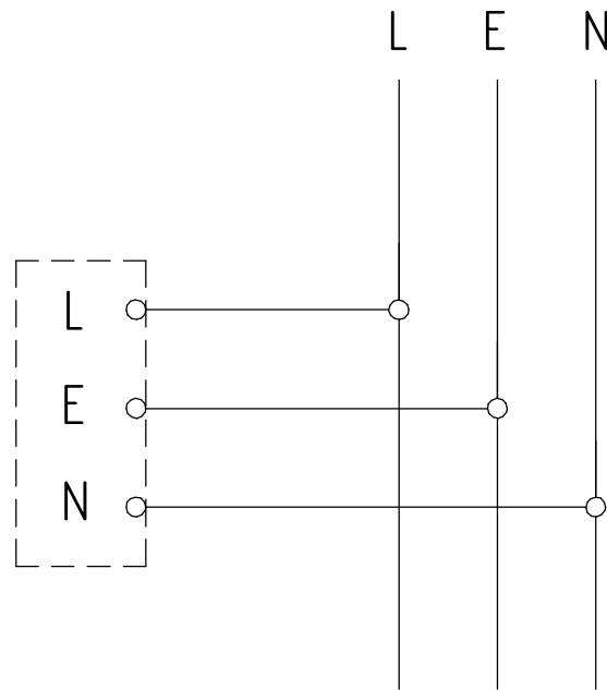
Рисунок 2 - Схема подключения к сети светильников ДКУ63
