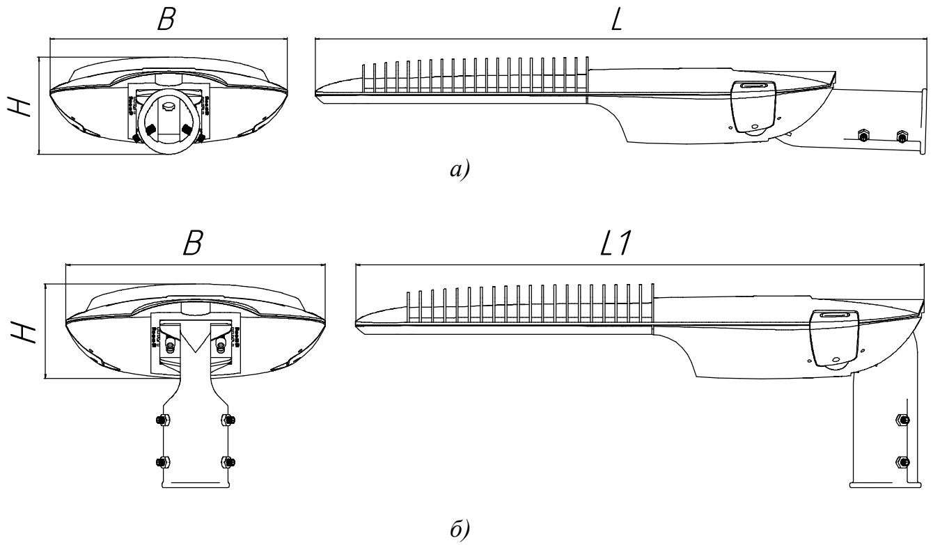
Рисунок 1 - Внешний вид и габариты светильников серии ДКУ63 (а - установка на Г-образный кронштейн; б - на торшерную опору).
