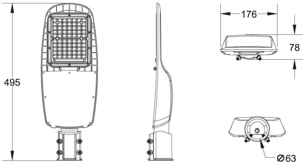
Рисунок 2 - Вид светильника ДКУ62-40-001, ДКУ62-60-001.
