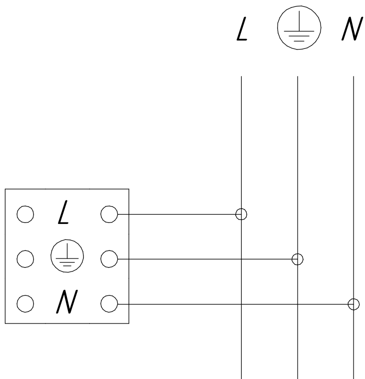
Рисунок 2 - Схема подключения светильников к сети
