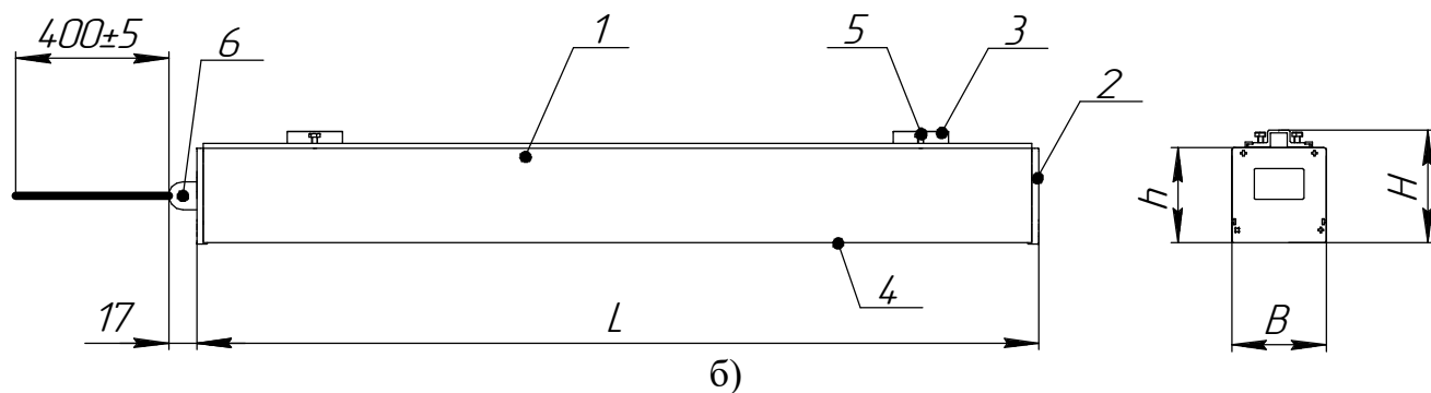
Рисунок 1 - Общий вид светильника серии ДСП45 Liner P HE 1 - корпус, со встроенным светодиодным модулем и источником питания, 2 - крышка, 3 - скоба подвеса, 4 - рассеиватель, 5 - винт М4, 6 - сальниковый ввод.
