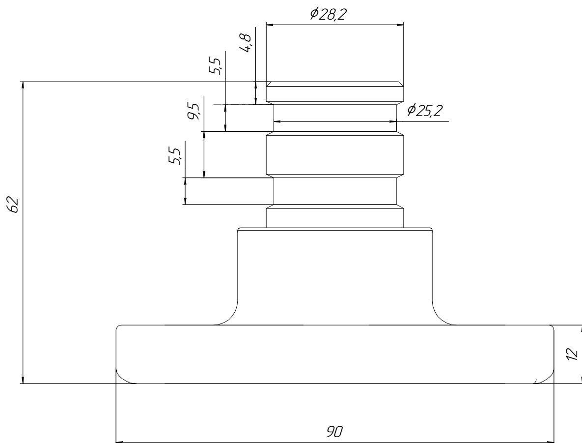
Рисунок 1 - Общий вид, габаритные размеры светильника ДБУ04-XX-X01.
