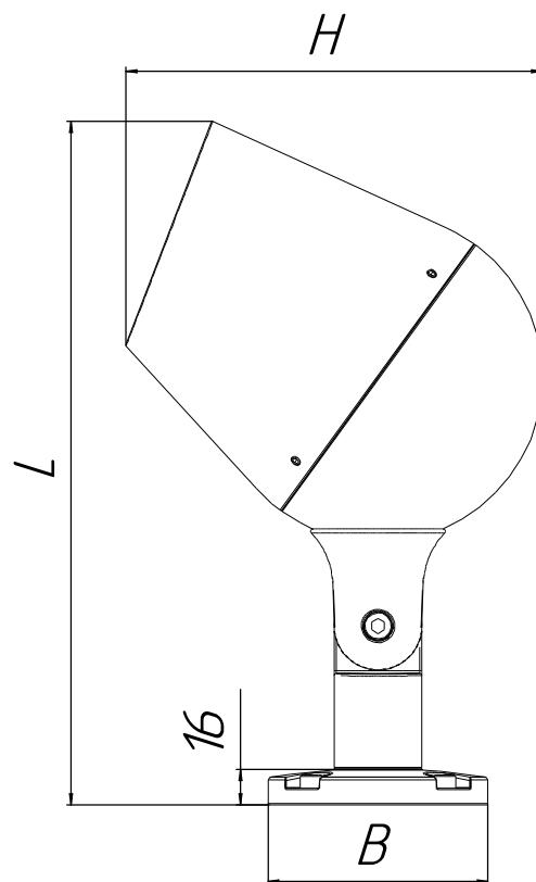
Рисунок 4а - Общий вид, габаритные размеры светильника ДБУ04-XX-X04.
