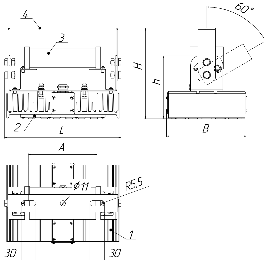
Рисунок 1а - Общий вид прожекторов мощностью 40, 80 Вт 1 - корпус, 2 - светодиодный модуль с линзами, 3 - источник питания (драйвер), 4 - узел крепления (лира).
