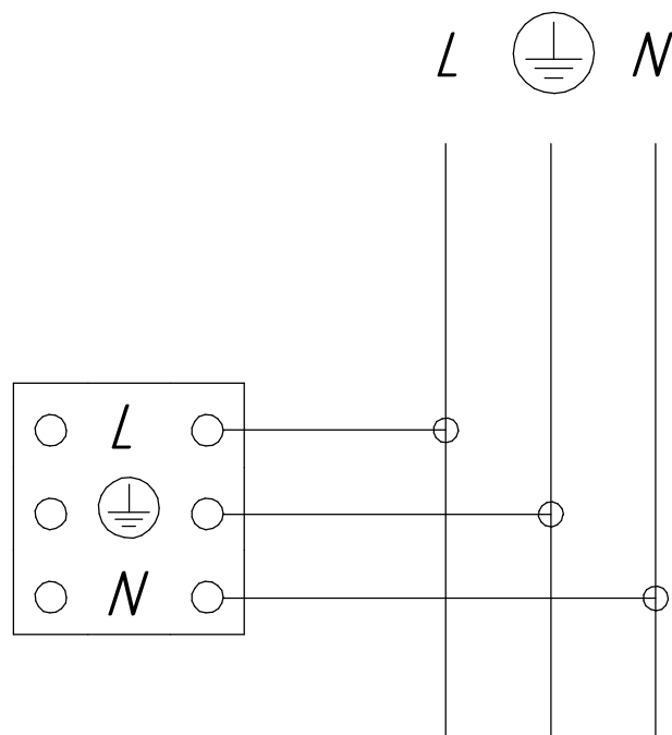
Рисунок 2а - Схема подключения прожекторов без управления
