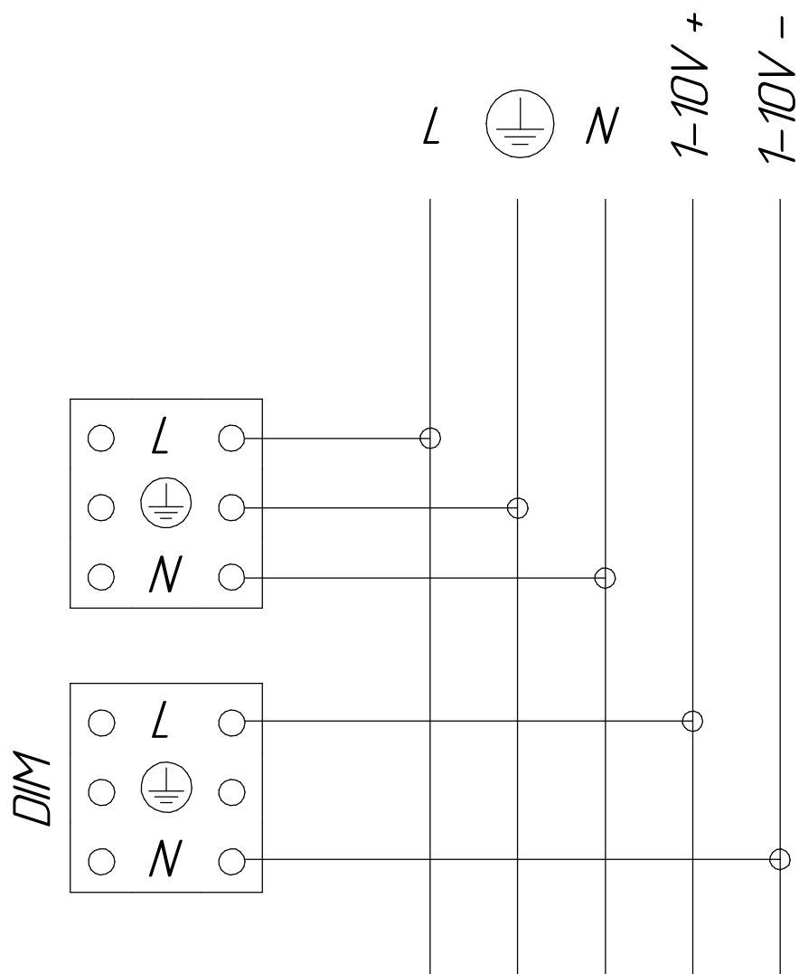
Рисунок 2б - Схема подключения прожекторов с управлением по протоколу 1-10 В
