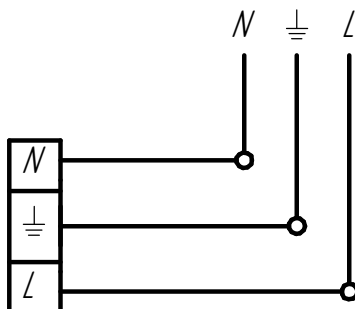
Рисунок 3 - Схема подключения светильника к сети
