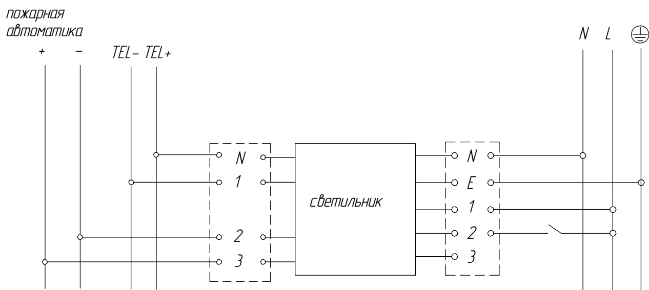
Рисунок 2 - Схема подключения светильника серии ДСП51 Leader EM к электрической сети
