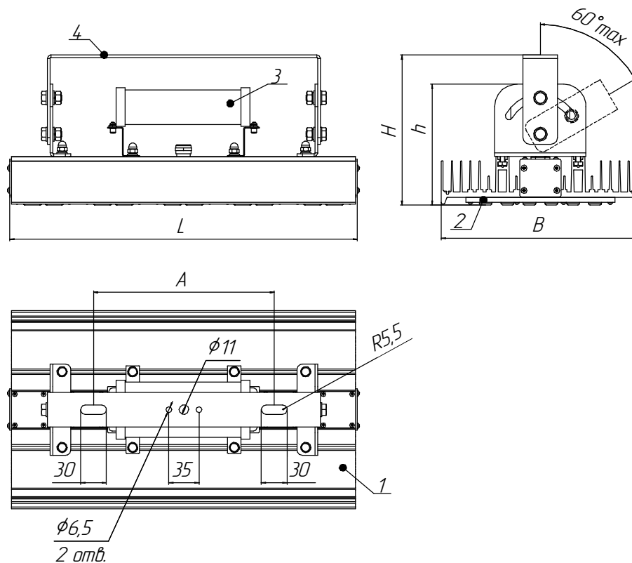
Рисунок 1б - Общий вид светильников мощностью 120, 160, 200, 240 Вт. 1 - корпус, 2 - светодиодный модуль с линзами, 3 - источник питания (драйвер), 4 - узел крепления (лира).
