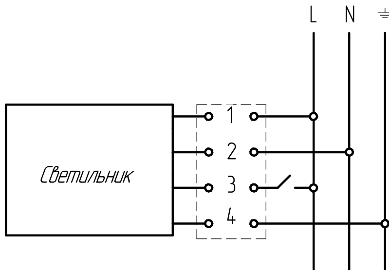
Рисунок 2 - Схема подключения светильника к сети 1 - не коммутируемая фаза 3 - коммутируемая фаза
