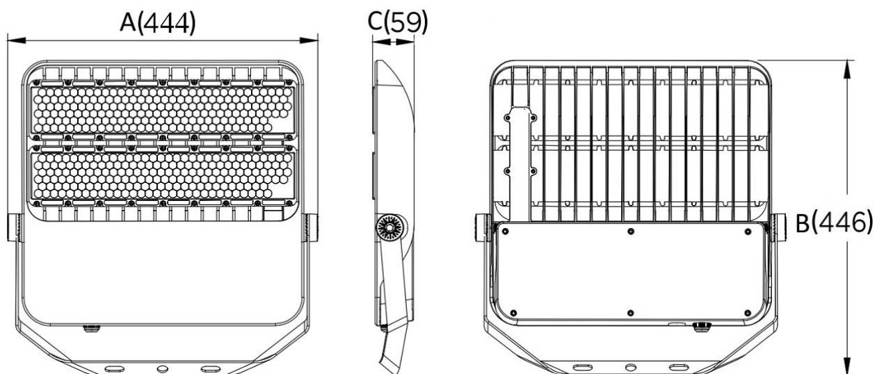
ДО17-240, ДО17-300, ДО17-400
