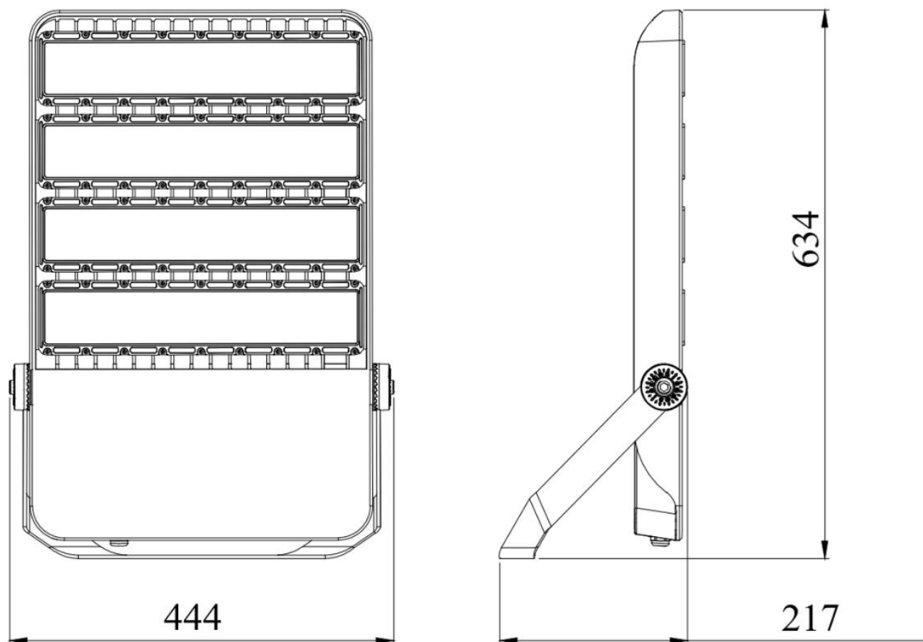
Рисунок 2в - Внешний вид и габаритные размеры прожекторов серии ДО17-600 в развернутом положении
