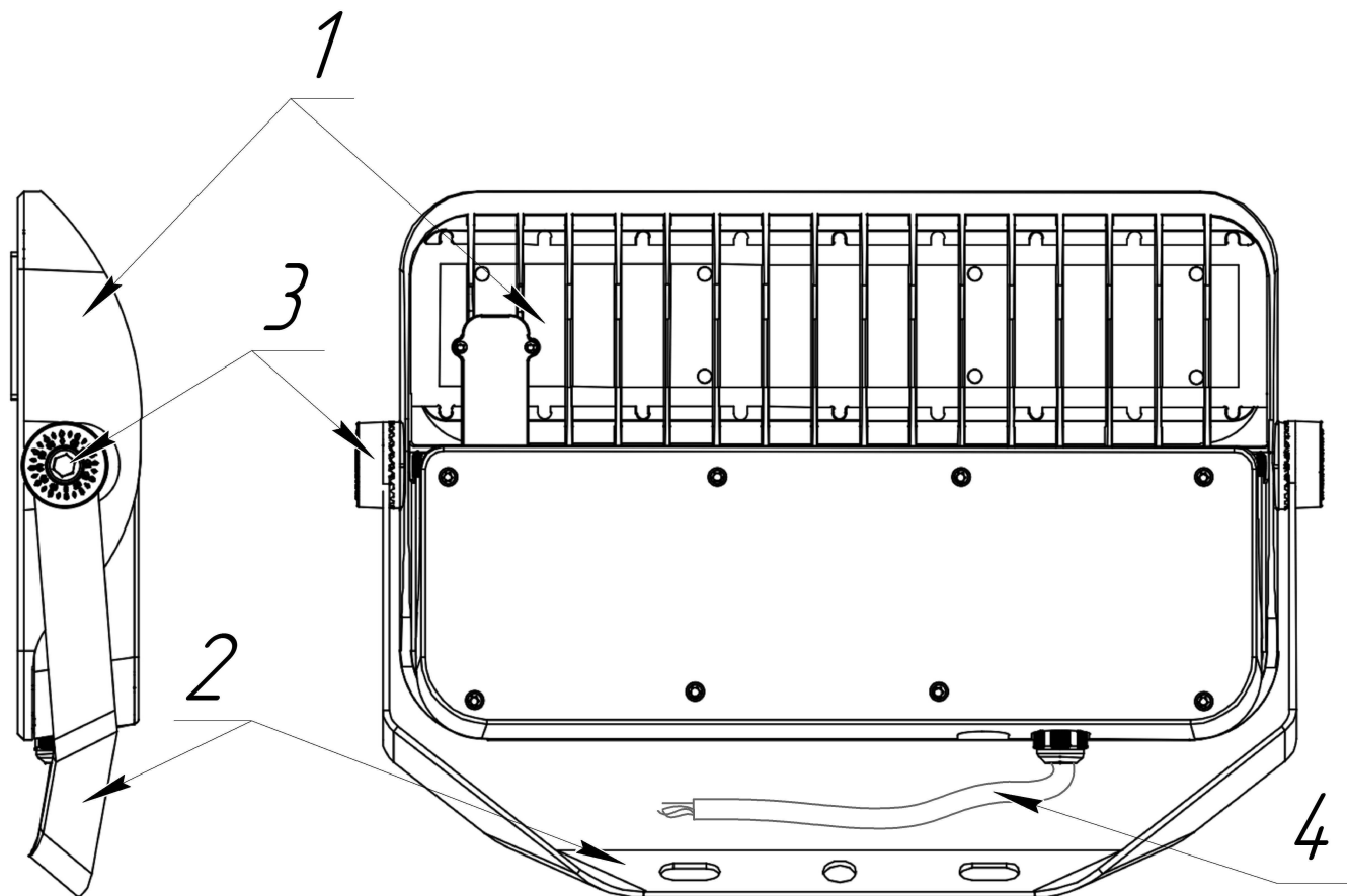
Рисунок 3 - Устройство прожектора серии ДО17
