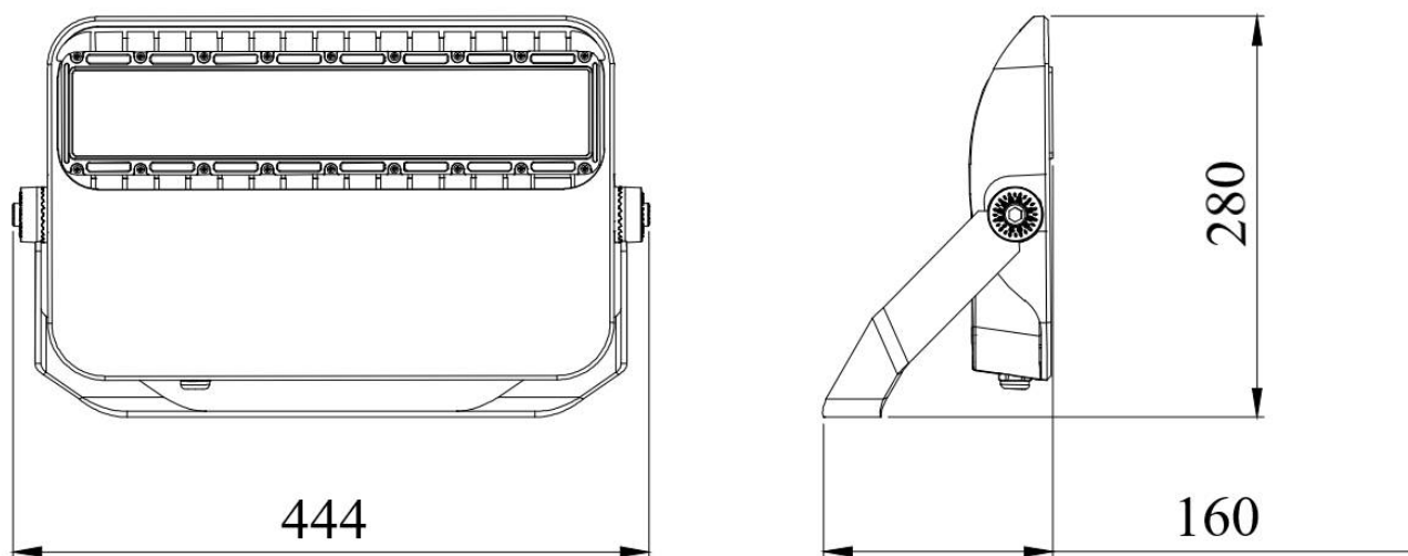
ДО17-100, ДО17-150, ДО17-200
