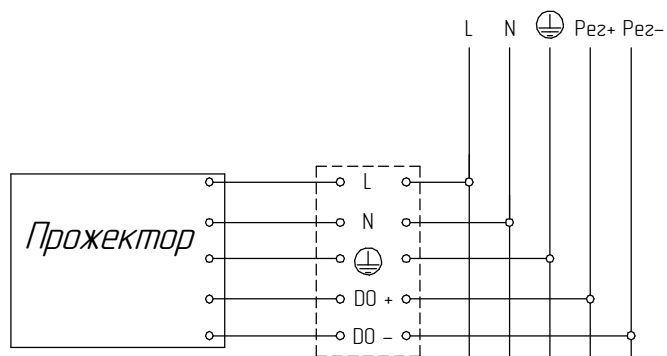
б) с управлением по протоколу 0-10В
