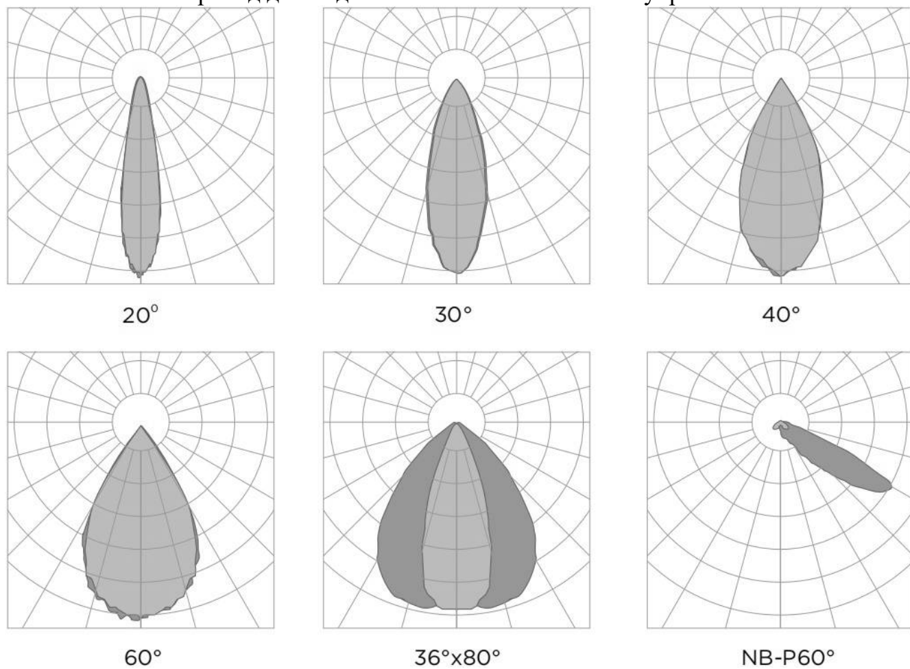
Рисунок 4 - Распределение света (КСС)
