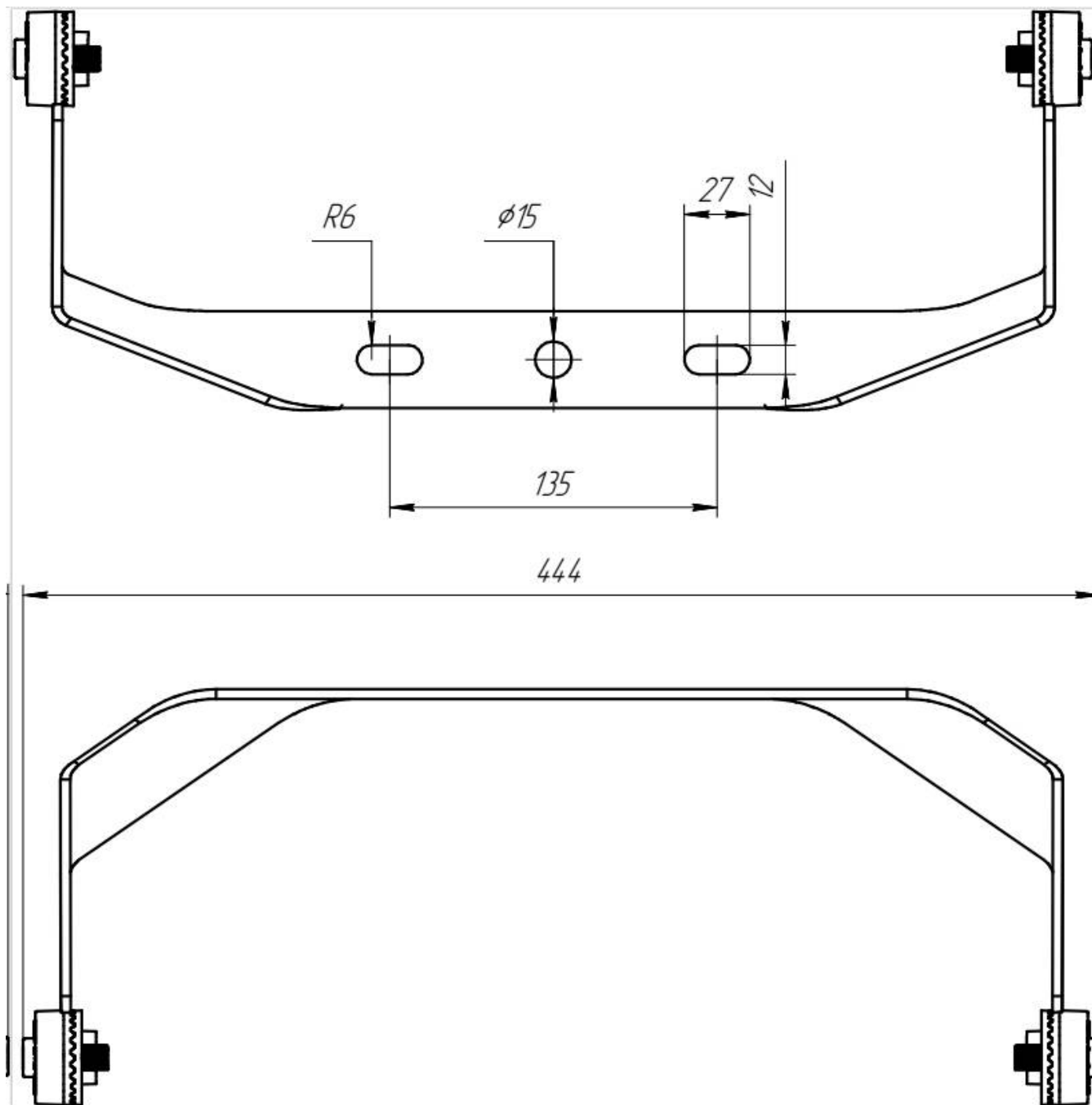
Рисунок 6 - Габаритные и установочные размеры лиры ДО17
