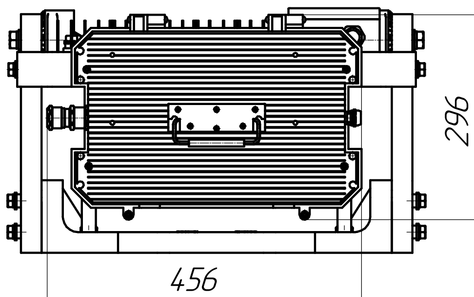
Рисунок 3 - Габаритные размеры отсека источника питания прожекторов ДО28
