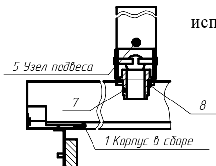
Способ установки светильника
