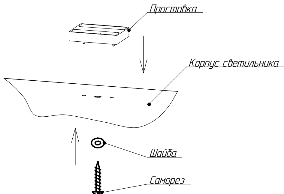
Рисунок 3 - Схема установки проставки пластиковой и крепления светильников
