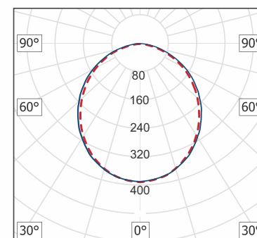
ДСО18-10 Profi I B4H4L50
