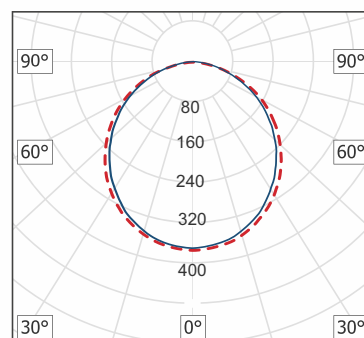
ДСО18-10 Profi I B5H5L50
