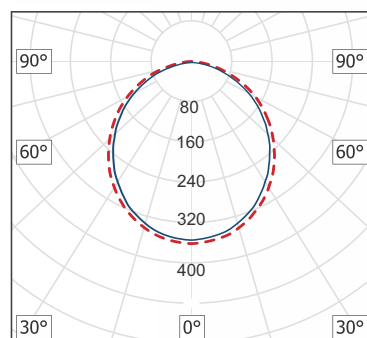
ДСО18-10 Profi I B3H9L50
