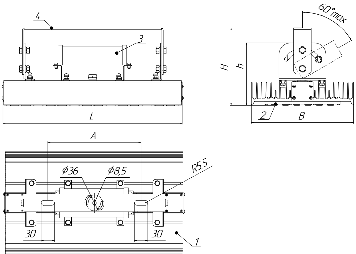
Рисунок 1б - Общий вид светильников мощностью 120, 160, 200, 240 Вт.
