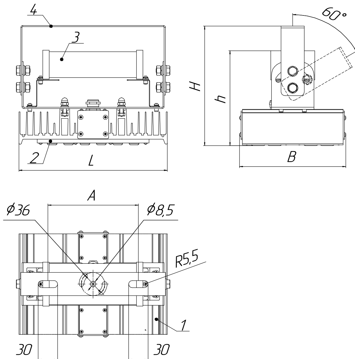
Рисунок 1а - Общий вид светильников мощностью 40, 80 Вт.
