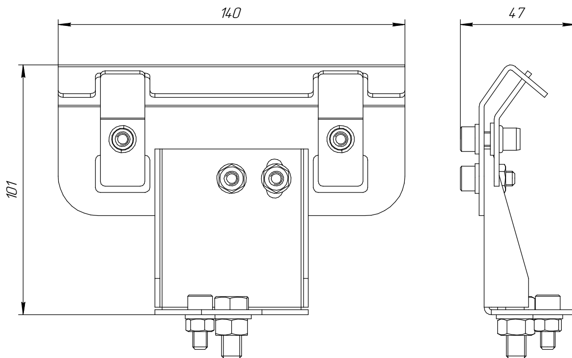
Рисунок 3 - Подвес на горизонтальный трос (для троса диаметром 6-12 мм).
