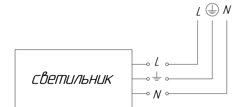
Рисунок 2 - Схема подключения светильников к сети
