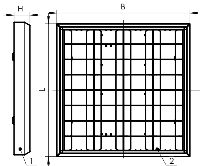
Рис. 1.1 ЛПО10-4x18 1. Корпус в сборе; 2. Решетка зеркальная
