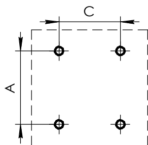
Рис. 2. Разметка расположения точек крепление светильника.
