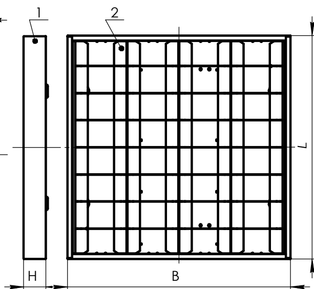
Рис. 1.3 ЛПО10-4x14 1. Корпус в сборе; 2. Решетка зеркальная
