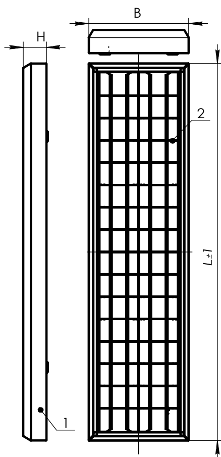
Рис. 1.2 ЛПО10-2x36 1. Корпус в сборе; 2. Решетка зеркальная
