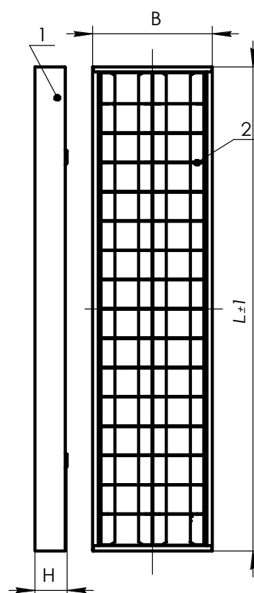
Рис. 1.3 ЛПО10-4x14 1. Корпус в сборе; 2. Решетка зеркальная
