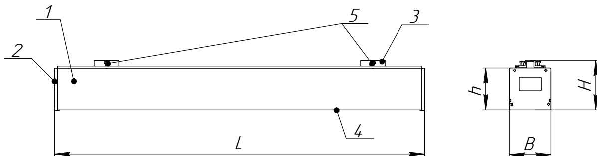
Рисунок 1 - Общий вид светильника серии ДСП45 Liner P. 1 - корпус, со встроенным светодиодным модулем и источником питания, 2 - крышка, 3 - скоба подвеса, 4 - рассеиватель, 5 - винт М4.
