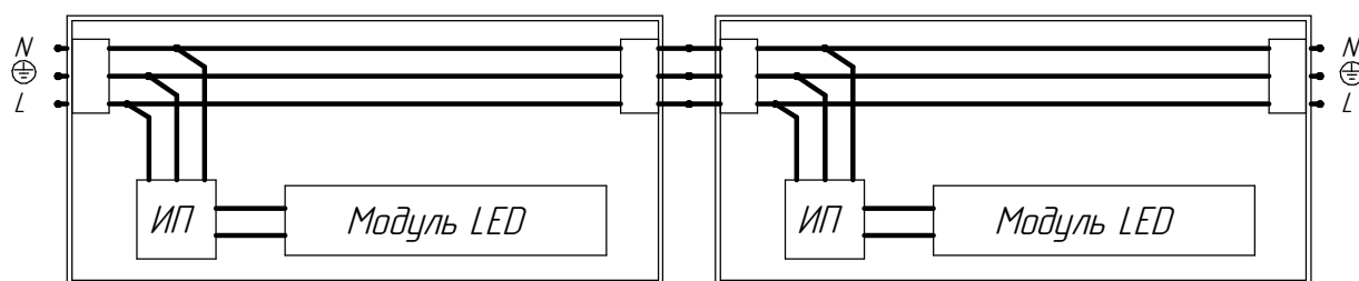
Рисунок 8 - Схема сквозной проводки
