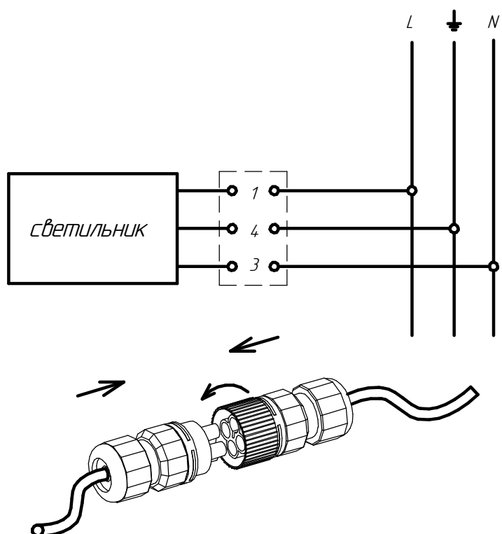
Рисунок 6 - Схема подключения светильника с магистральной проводкой
