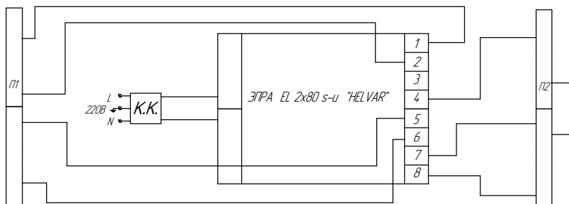
Рисунок 12. ЛСО02-2x80 Universal, схема электрическая с ЭПРА
