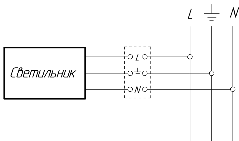
Схема подключения светильника к сети
