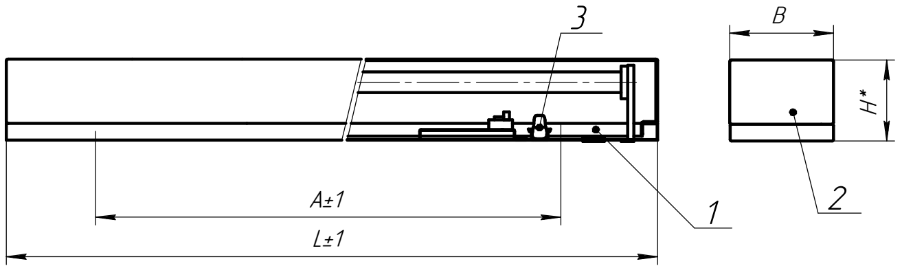
Рисунок 1. ЛПО46-18; 36; 2x18; 2x36 1. корпус в сборе; 2. рассеиватель; 3. защелка
