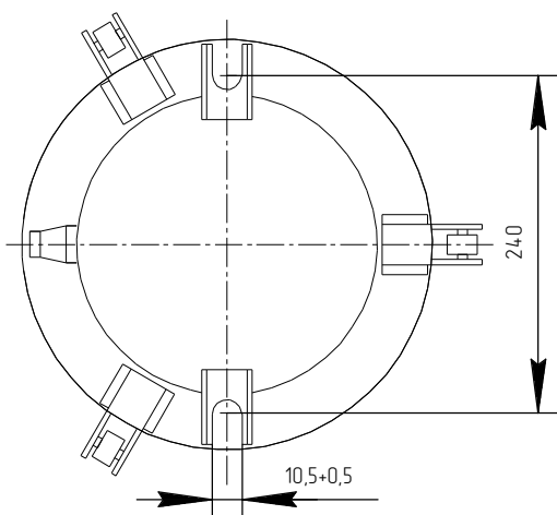
Рисунок 4. - установочные размеры.
