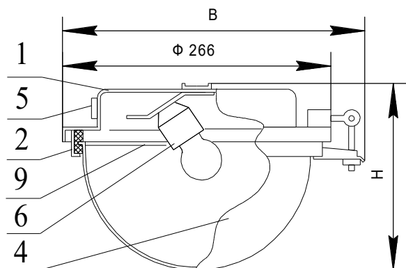
Рисунок 1. НПП03-60, 100-001; НПП03-100-002: 1.Корпус в сборе; 2.Кольцо в сборе; 4.Рассеиватель; 5.Садовый ввод или заглушка; 6.Патрон; 9.Экран.
