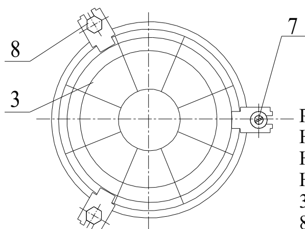
Рисунок 1. НПП03-60, 100-001; НПП03-100-002: 1.Корпус в сборе; 2.Кольцо в сборе; 4.Рассеиватель; 5.Садовый ввод или заглушка; 6.Патрон; 9.Экран.
