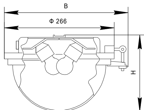
Рисунок 2. НПП03-2х40-001, НПП03-2х40-002.
