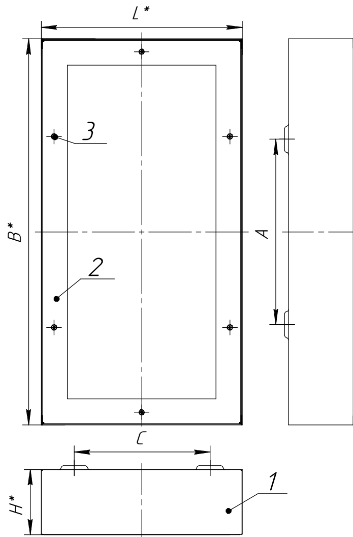
Рисунок 1: 1. Корпус в сборе, 2. Обечайка в сборе. 3. Винт
