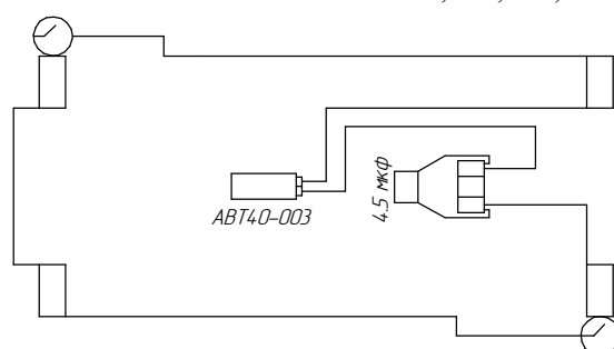
Схема электрическая (компенсированная) на светильники ЛПО15-2х18-021;022;121;122
