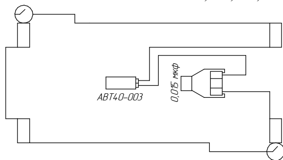
Схема электрическая (не компенсированная) на светильники ЛПО15-2х18-001;002;101;102
