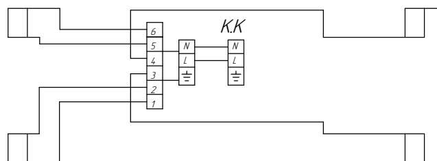
Схема электрическая с аппаратом ЛПО15-2х18-031;032;131;132
