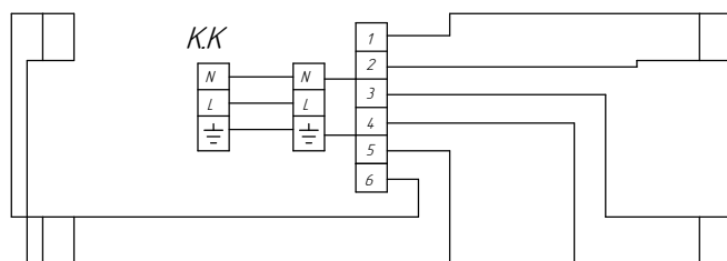
Схема электрическая на светильники ЛПО15-2х18-011;012;111;112
