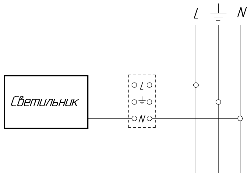
Рис.3 Схема подключения светильника к сети.
