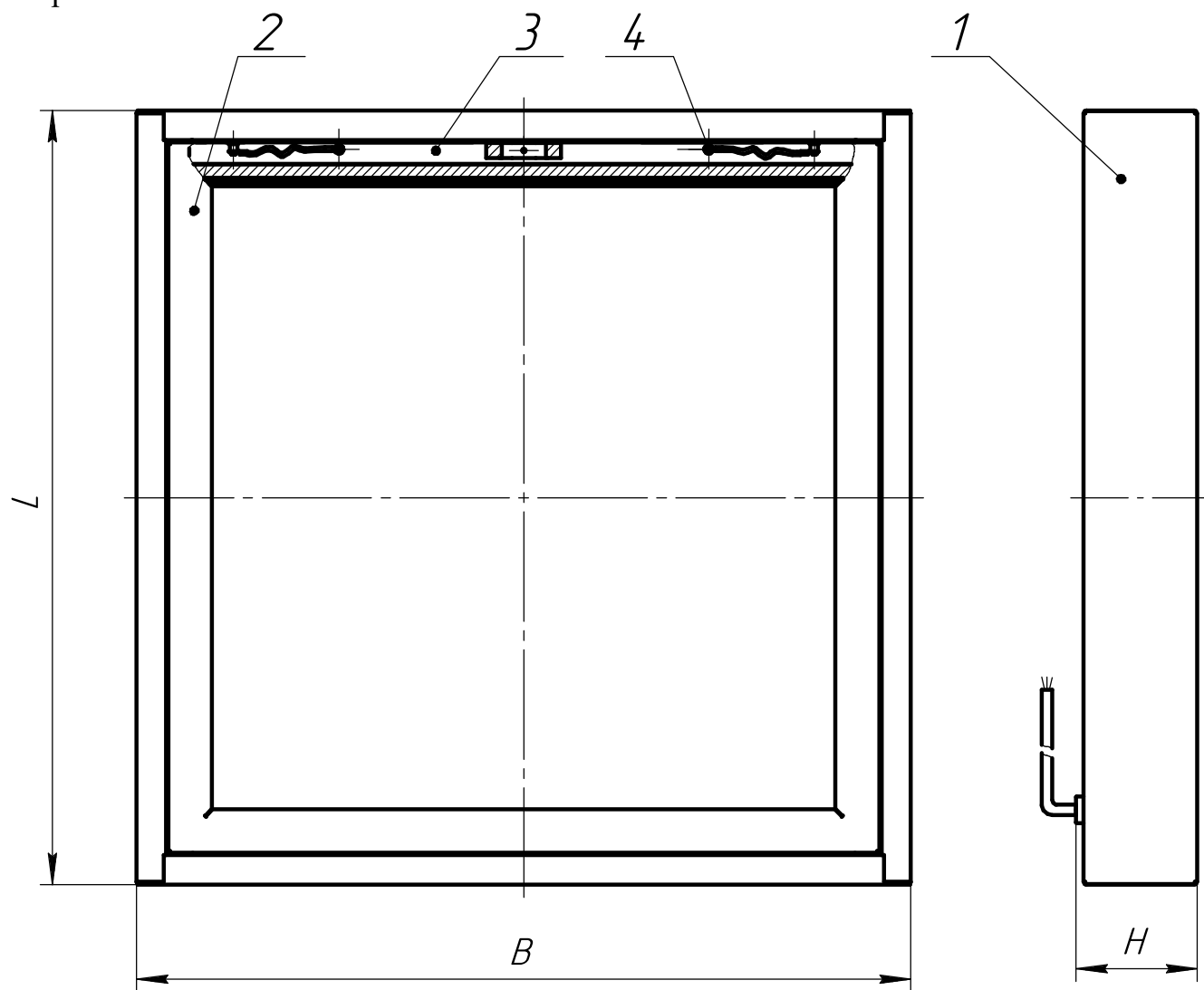
Рис.1 Общий вид светильника.
