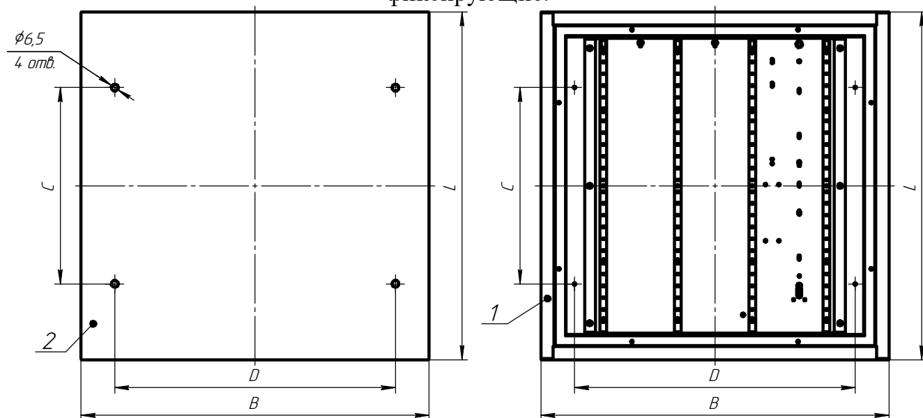
Рис.2. Разметка установочных отверстий под светильник
