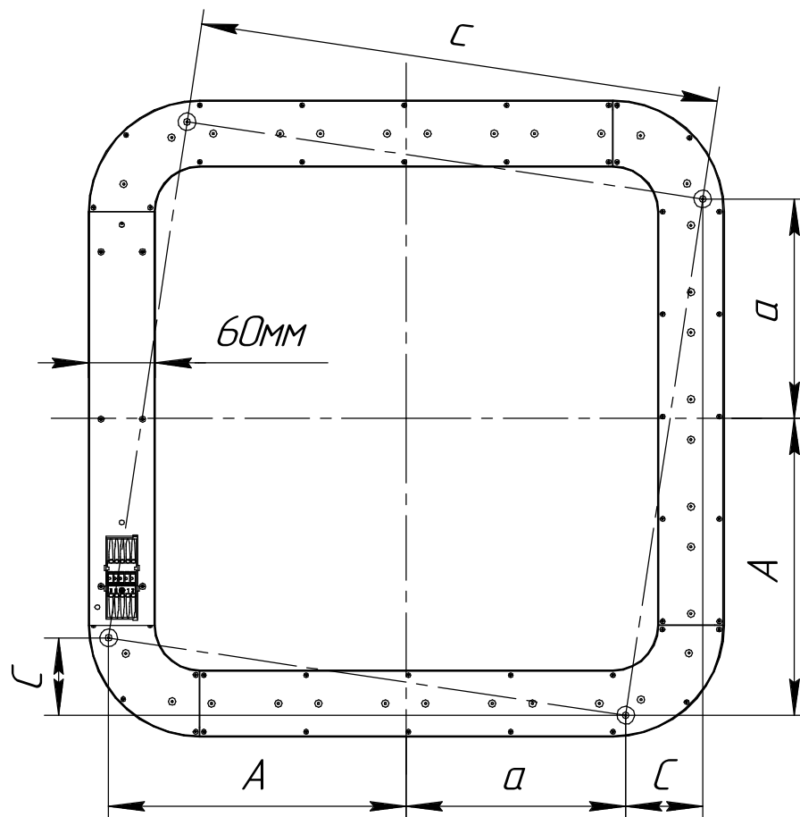
Рисунок 3 - Схема нанесения разметки для установки подвесов светильника Horizon Four Frame.
