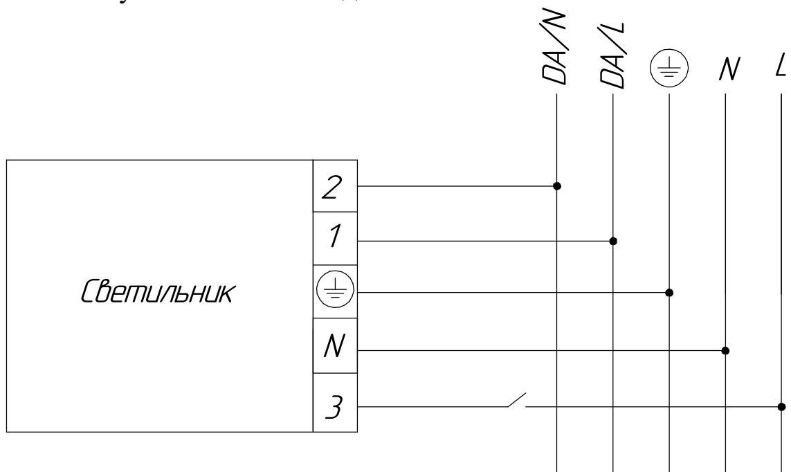
Рисунок 5 - Схема подключения светильника к сети
