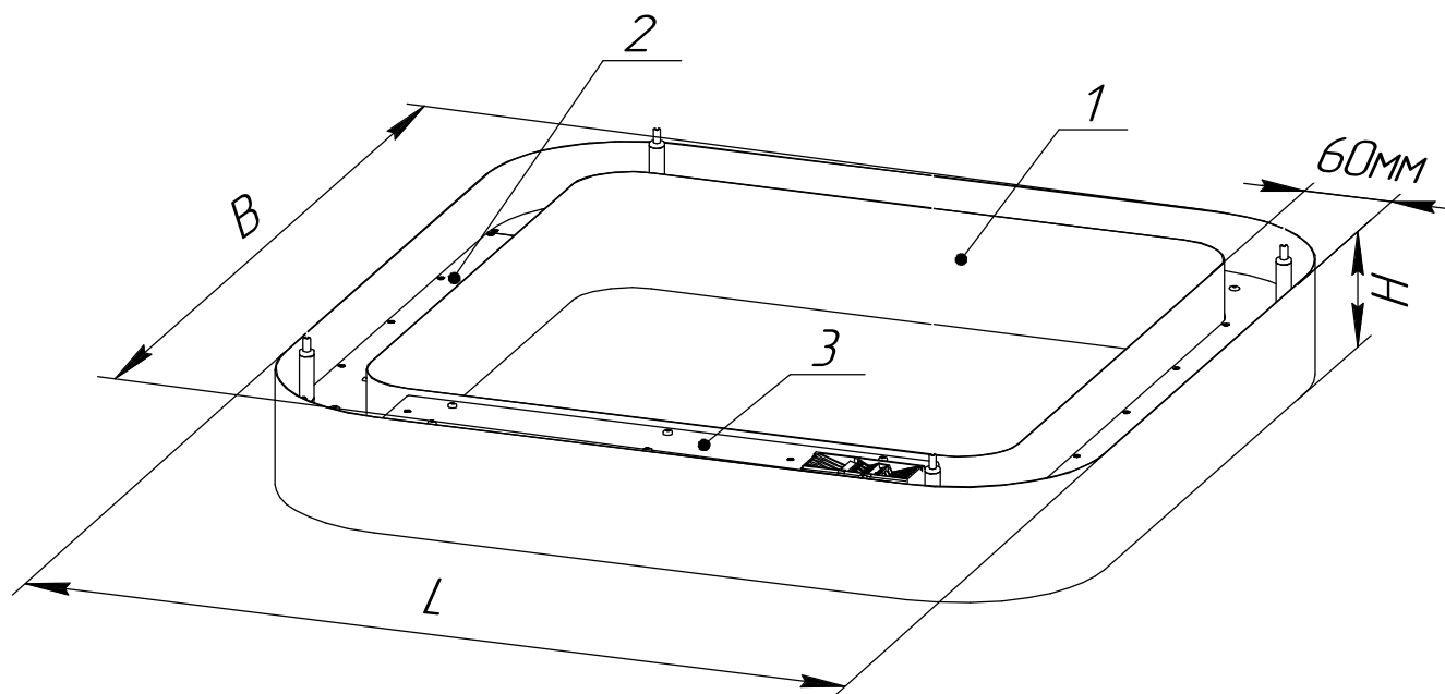
Рисунок 1 - Светильник серии ДСО33 Horizon Four Frame
