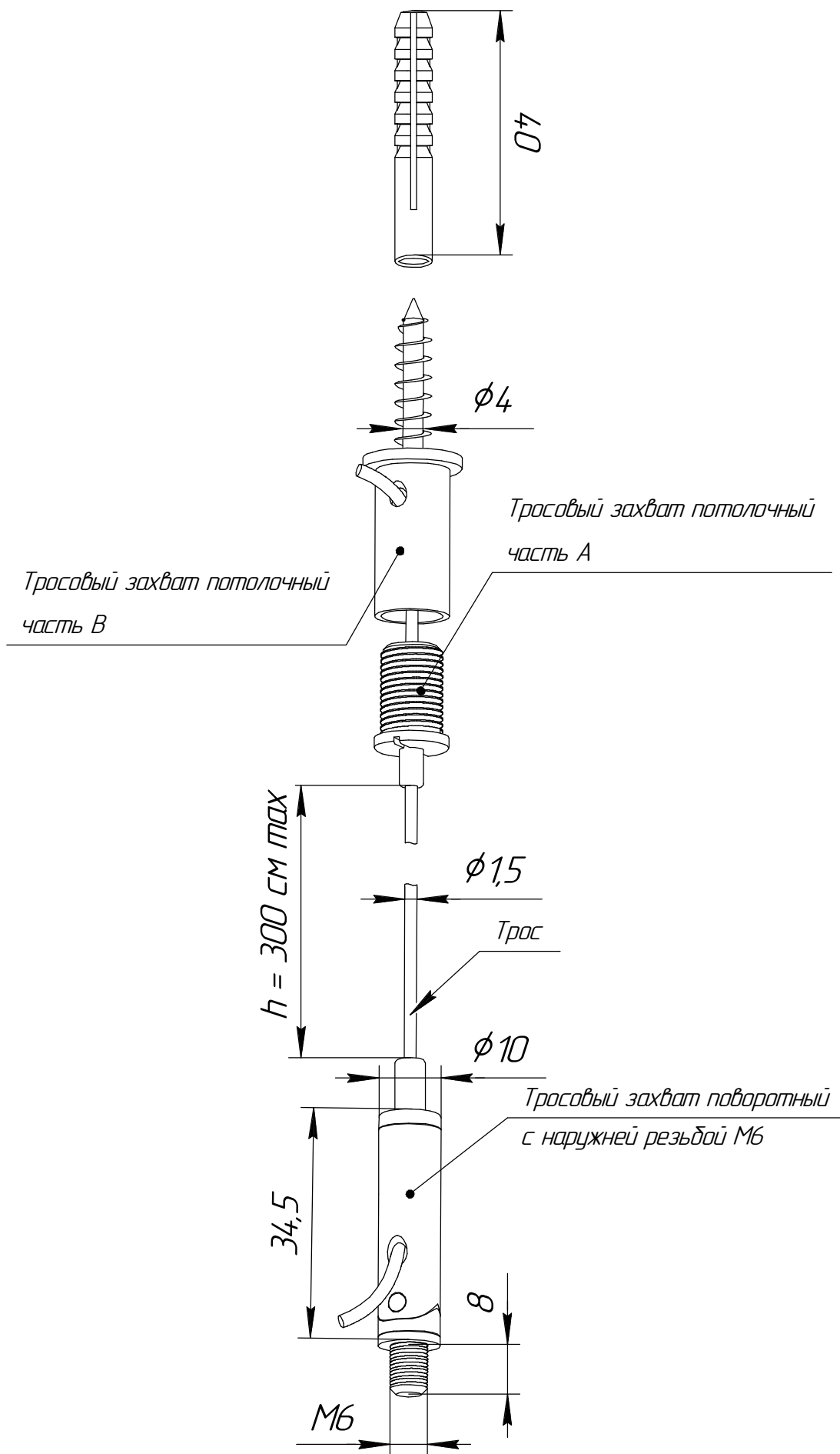
Рисунок 4 - Сборка тросового подвеса
