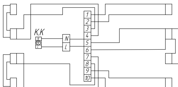
Схема электрическая на светильники ЛПО15-4х18-011,012;111;112
