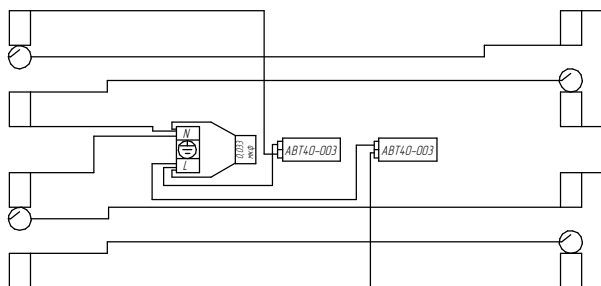
Схема электрическая (не компенсированная) на светильники ЛПО15-4х18-001,002;101;102
