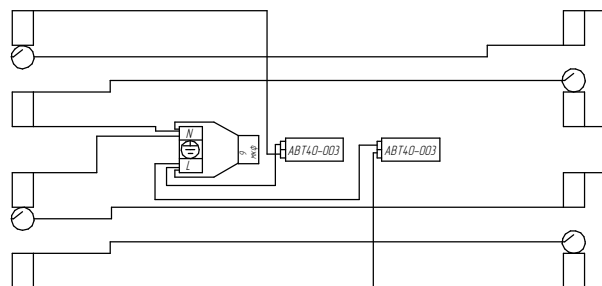
Схема электрическая (компенсированная) на светильники ЛПО15-4х18-021,022;121;122
