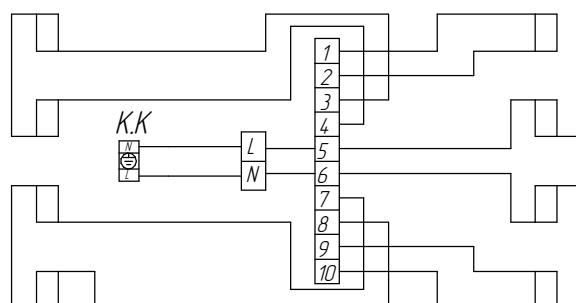
Схема электрическая с аппаратом ЛПО15-4х18-031,032;131;132
