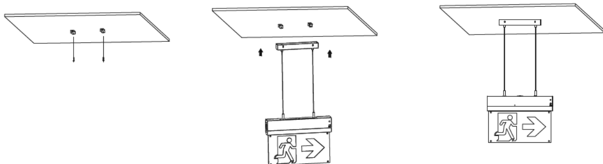
Рисунок 11 - Крепление на тросовых подвесах
