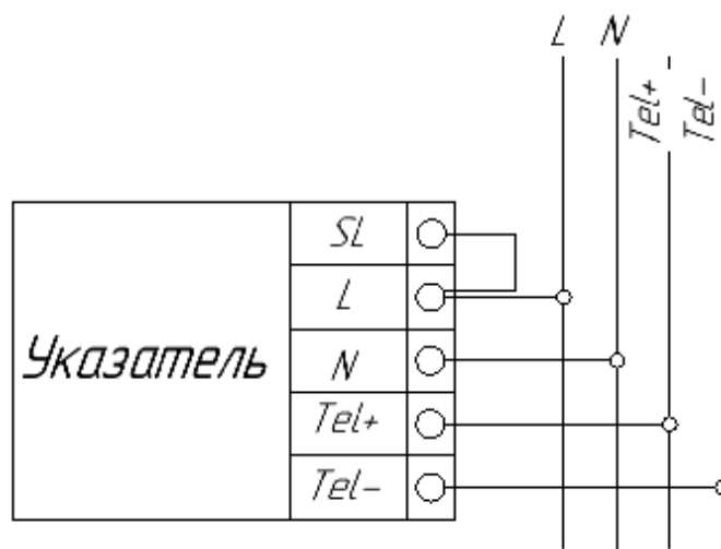
Рисунок 19 - Схема подключения указателя с функцией дистанционного тестирования к сети
