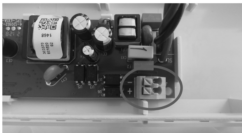
Рисунок 19а - Клемма подключения указателя с функцией дистанционного тестирования к сети
