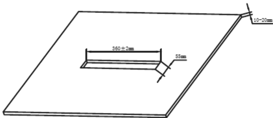
Рисунок 12 - Монтажное отверстие
