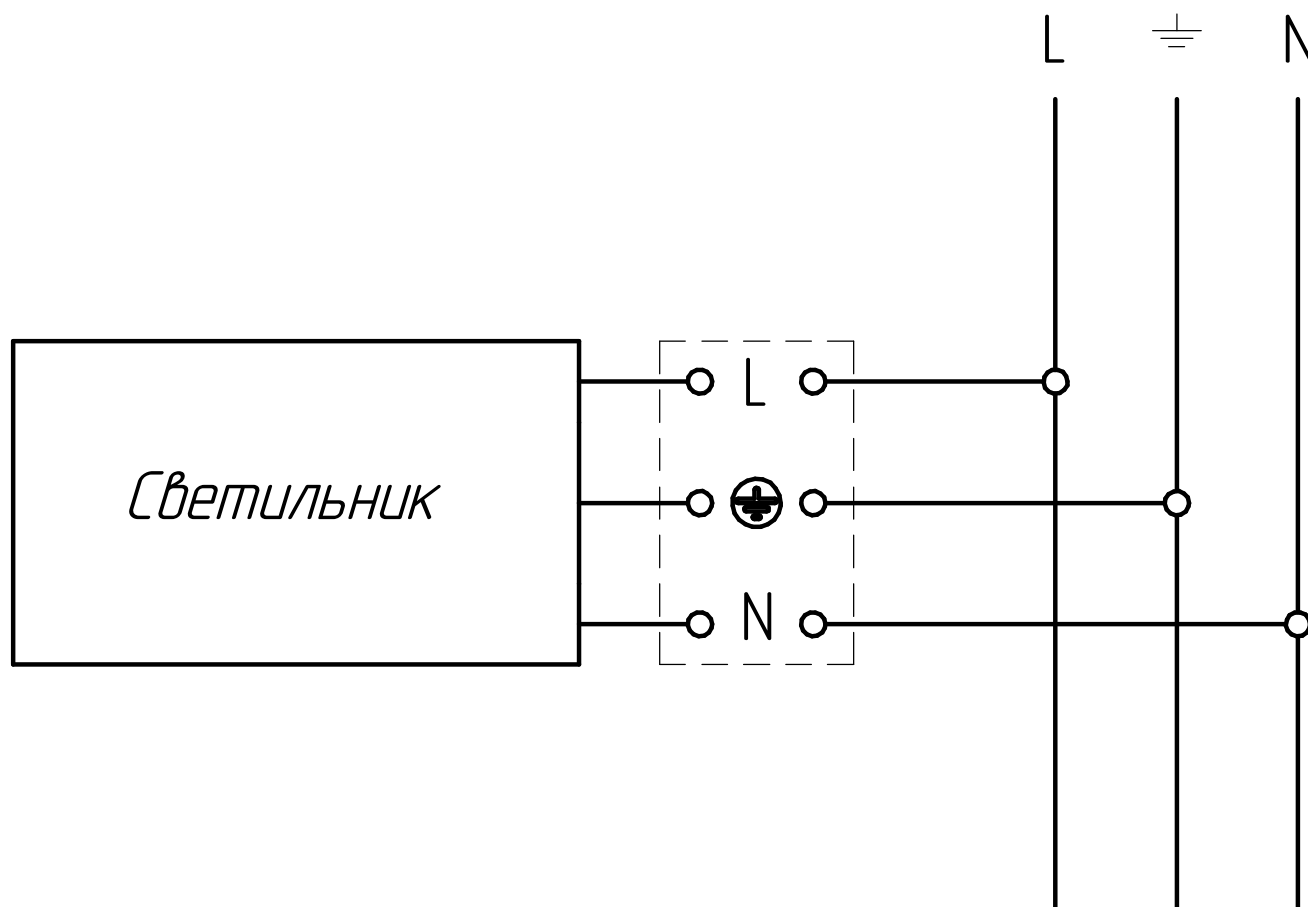
Рисунок 2 - Схема подключения светильника к электрической сети
