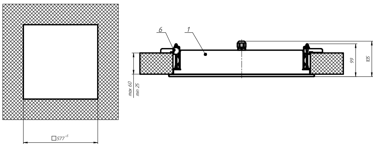
Рис.2.1 Установка светильника.
