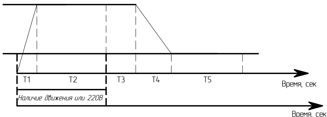
Рисунок 7 - График работы светильника с функцией Дежурный режим от датчика или выключателя
