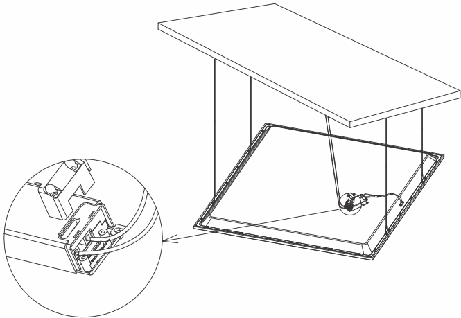
Подвесной монтаж
