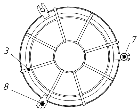
Рисунок 1в - ДПП03
