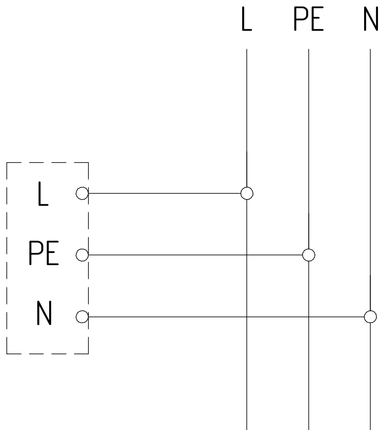
Рисунок 4 - Схема подключения светильника к сети
