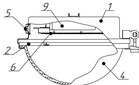
Рисунок 1б - ДПП03
