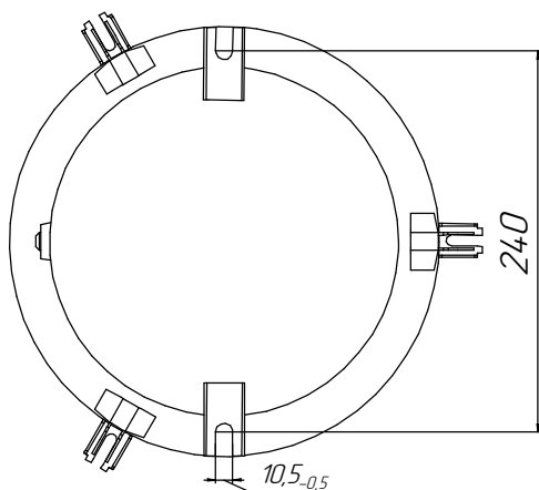
Рисунок 2 - Установочные размеры
