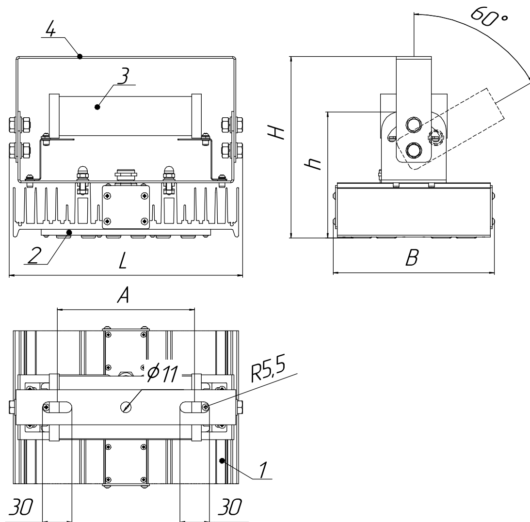
Рисунок 1а - Общий вид светильников мощностью 40, 80 Вт.
