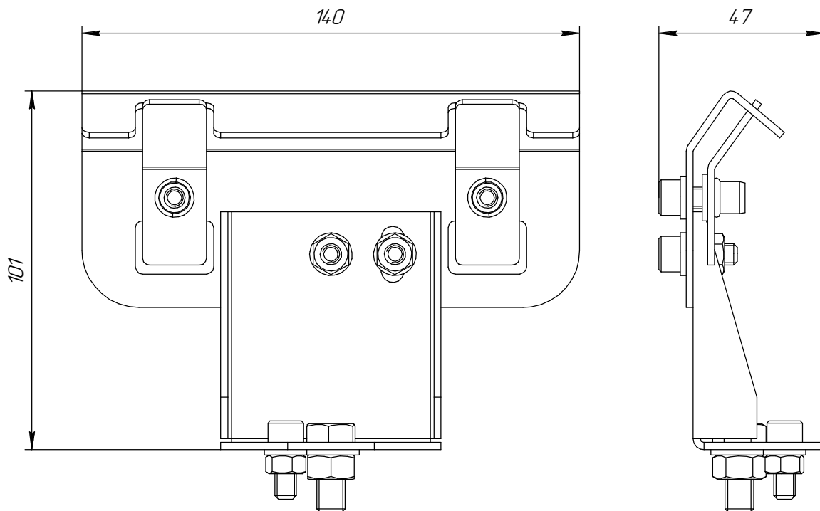
Рисунок 14 - Подвес на горизонтальный трос (для троса диаметром 6-12 мм).
