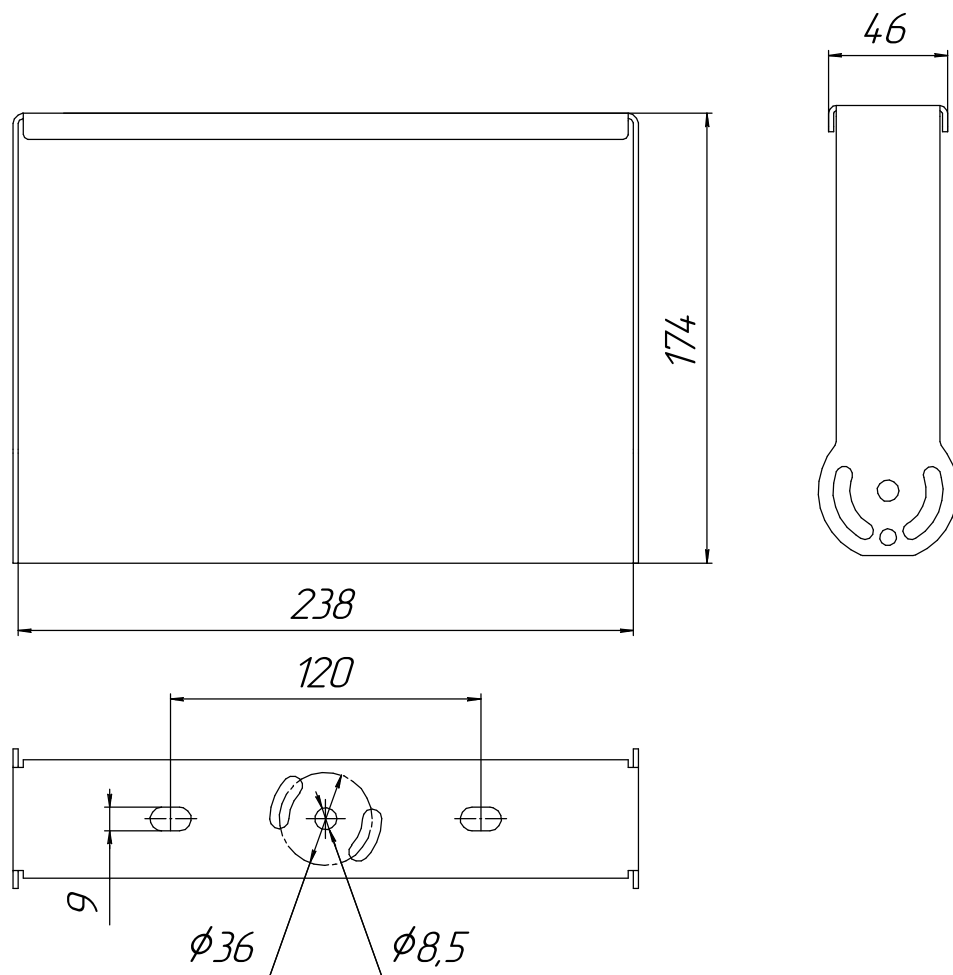
Рисунок 10 - Лира 745361027.
