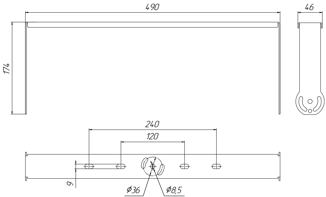
Рисунок 12 - Лира 745361027-02.
