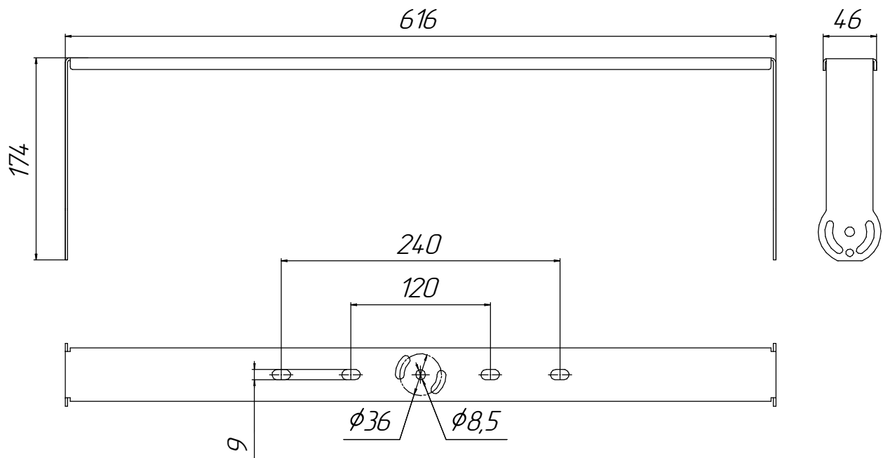
Рисунок 13 - Лира 745361027-03.
