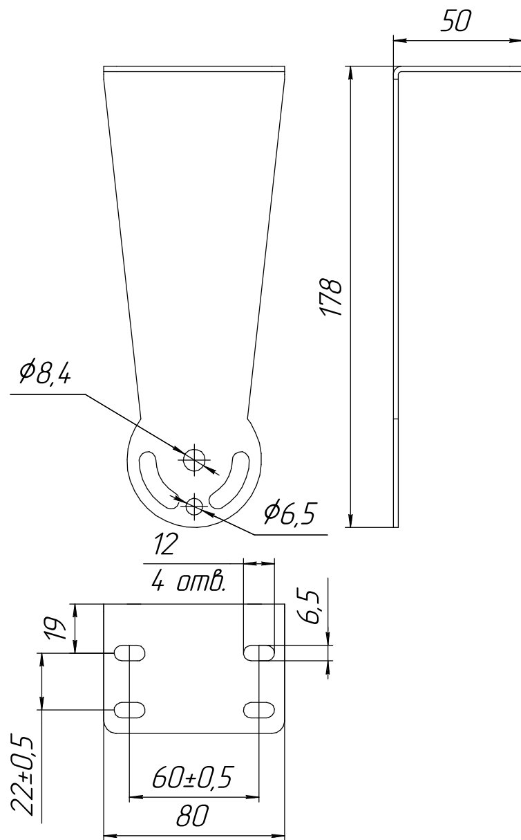
Рисунок 8 - Кронштейн 734313039.
