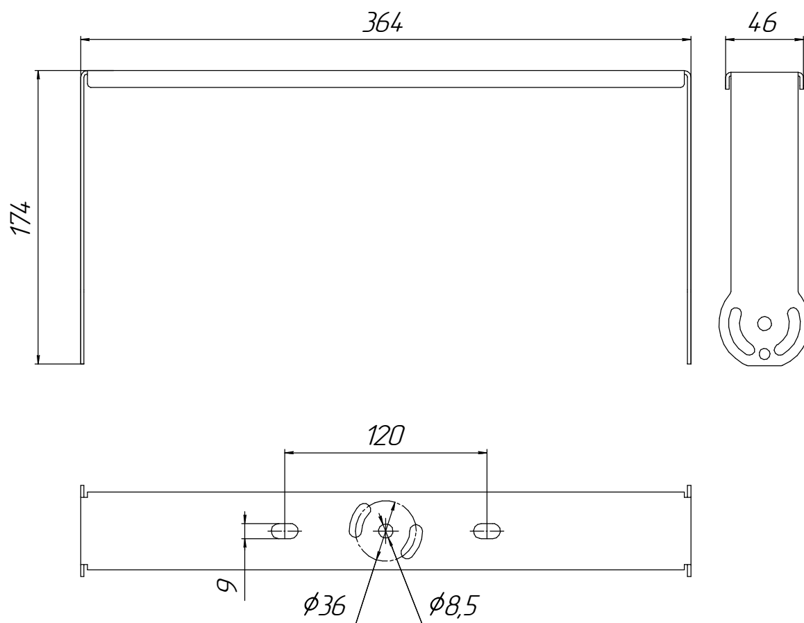
Рисунок 11 - Лира 745361027-01.
