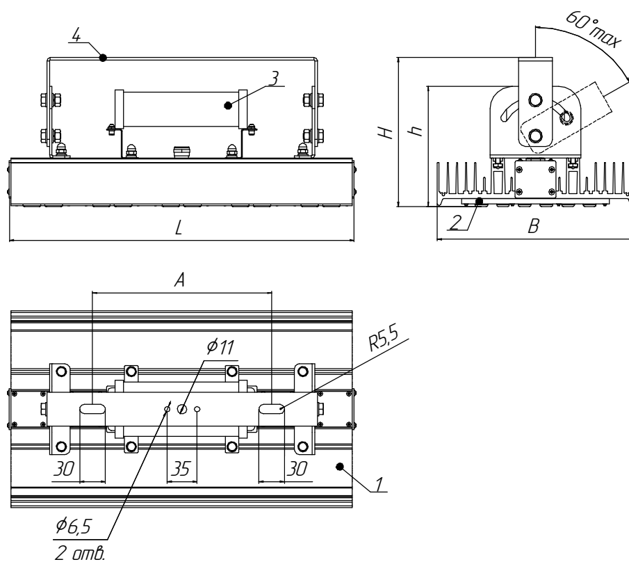
Рисунок 1б - Общий вид прожекторов мощностью 120, 160, 200, 240 Вт 1 - корпус, 2 - светодиодный модуль с линзами, 3 - источник питания (драйвер), 4 - узел крепления (лира).
