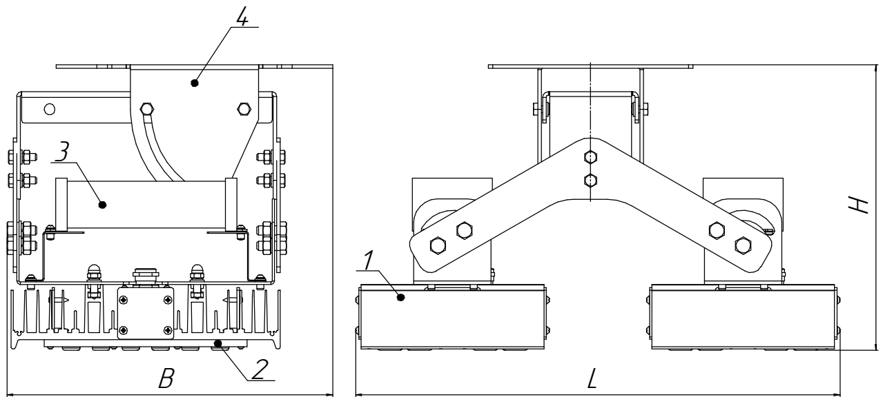
Рисунок 1в - Общий вид прожекторов мощностью 2х40, 2х80 Вт 1 - корпус, 2 - светодиодный модуль с линзами, 3 - источник питания (драйвер), 4 - узел крепления (лира).
