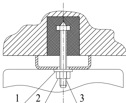
Рисунок 5. - крепление светильника на горизонтальную поверхность:
