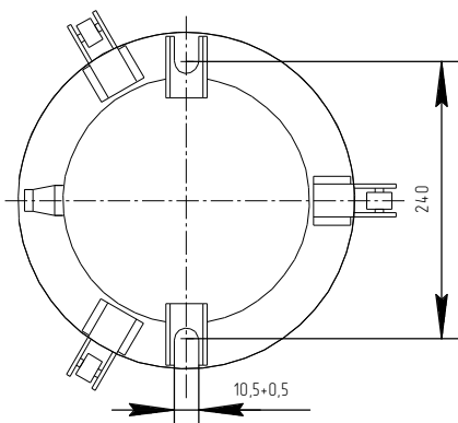
Рисунок 4. - установочные размеры.
