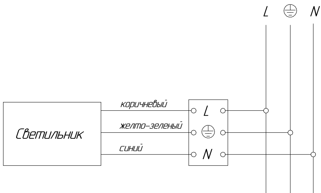
Рисунок 4 - Схема подключения к сети светильников
