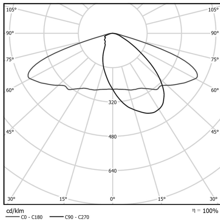
Рисунок 5 - КСС типа III
