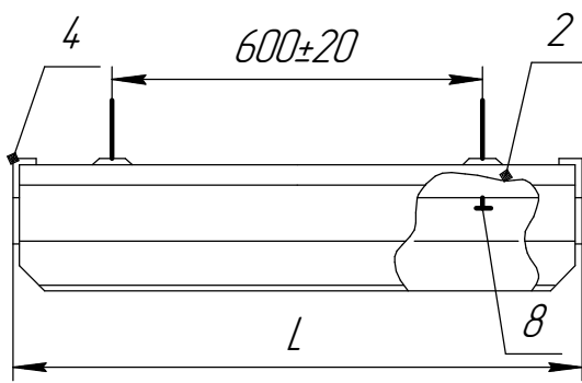
Рисунок 1: 1. Узел подвеса; 2. Корпус; 3. Отражатель; 4. Крышка торцевая; 5. Скоба с патронами; 8. Винт специальный.
