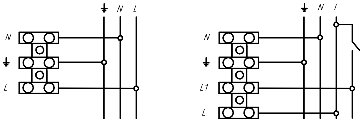
Рисунок 2 - Схема подключения светильника к сети (L -фаза, L1-коммутируемая фаза, N -нейтраль)
