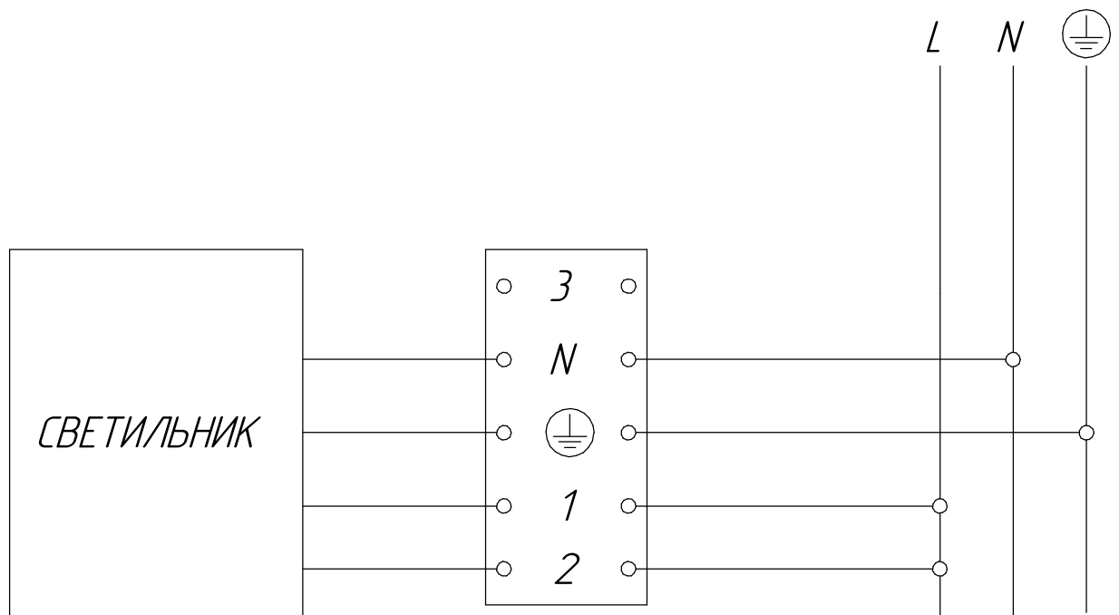
Рисунок 4 - Схема подключения светильников к сети 1 - питание светодиодных модулей, 2 - питание лампы.
