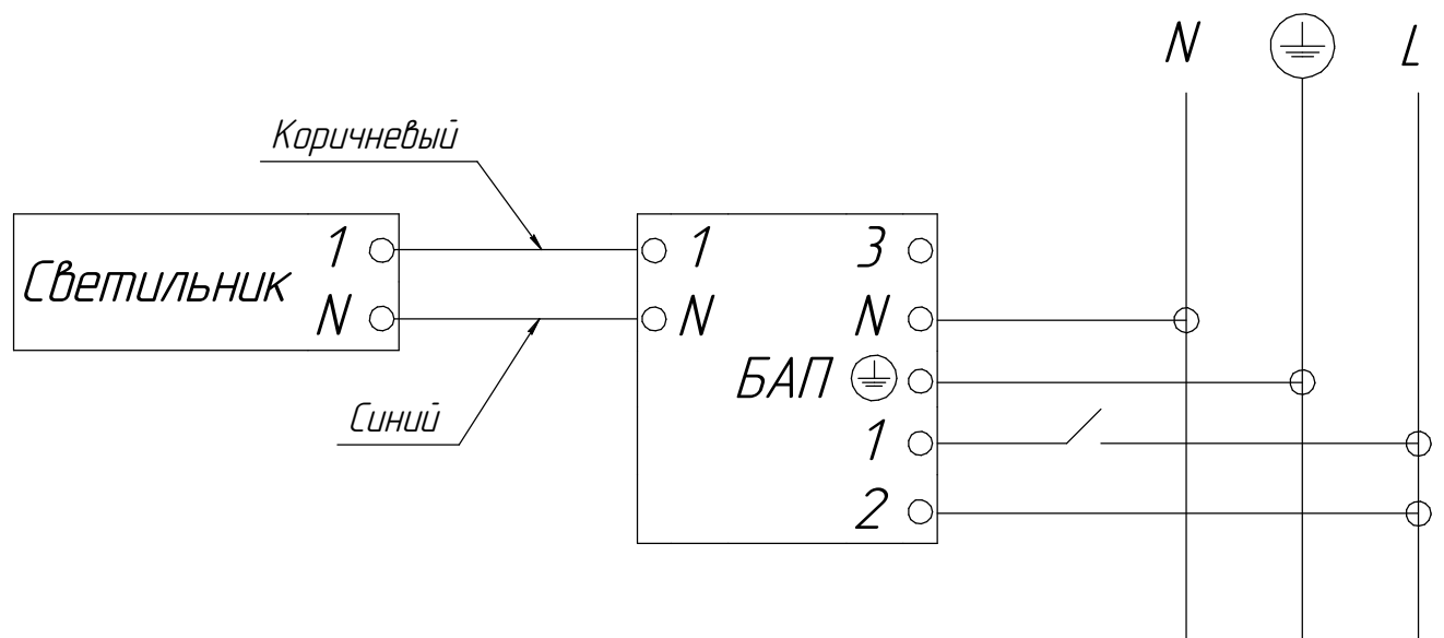
Рисунок 2б - Схема подключения светильников ДБО85 Sever EM1 к сети
