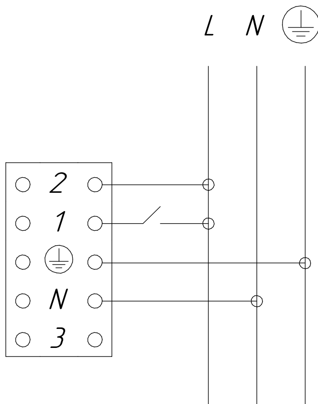
Рисунок 2а - Схема подключения светильников ДБО85 Tablette EM1 к сети
