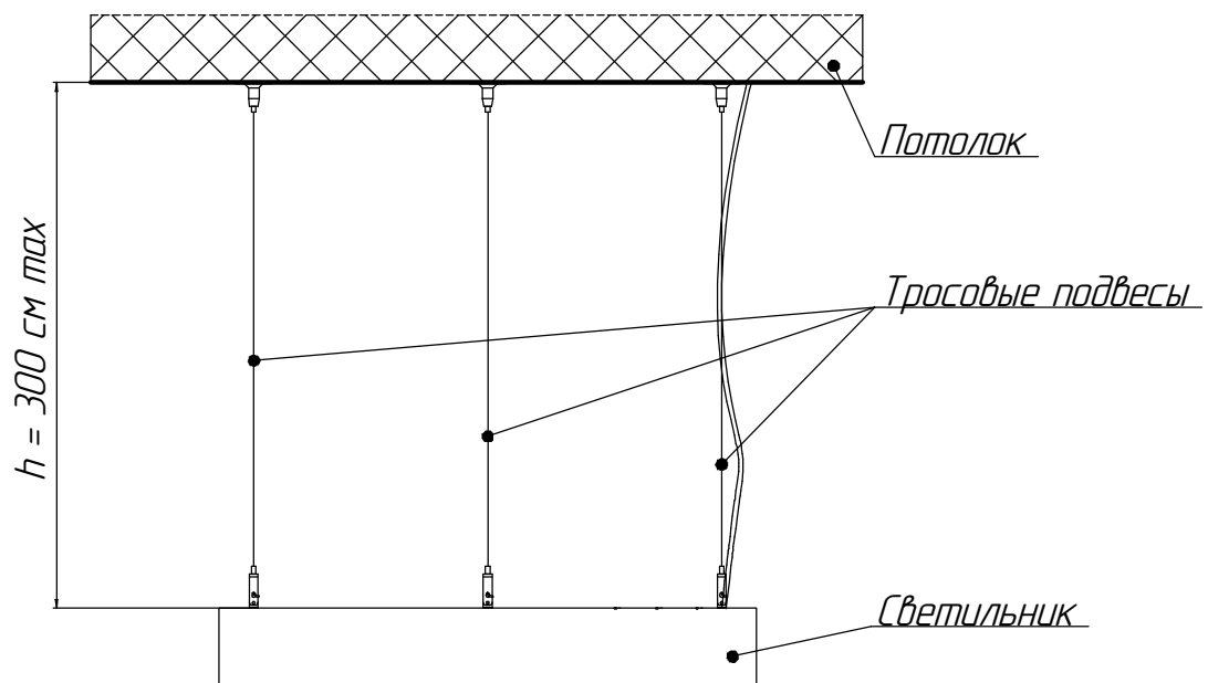
Рисунок 4 - Схема установка светильников.
