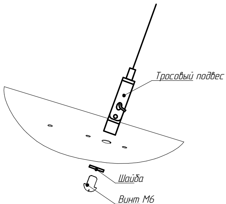
Рисунок 4 - Схема установки тросового подвеса
