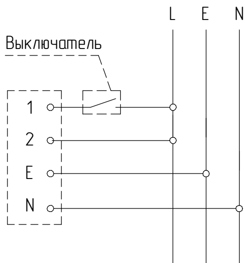
Рисунок 6 - Схема подключения светильников к сети 2 - некоммутируемая фаза, 1 - коммутируемая фаза
