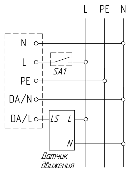
б) с датчиком движения
