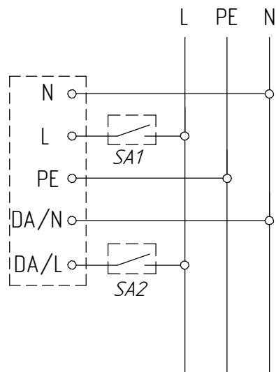
а) с выключателем
