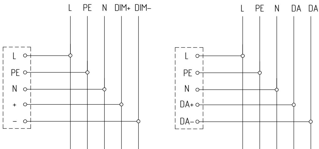
а) управление по протоколу 1-10V б) управление по протоколу DALI Рисунок 4 - Схема подключения светильников с управлением к сети
