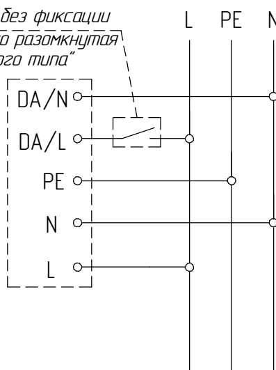
Рисунок 6 - Схема подключения светильников с функцией Диммирование Касанием к электрической сети
